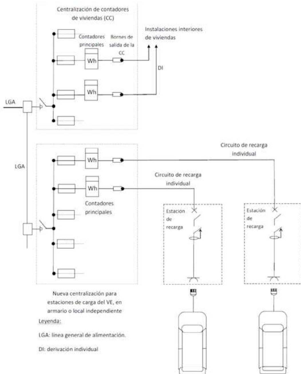
Figura 37. Esquema 3b de instalación individual con un contador principal para cada estación de recarga, con una nueva centralización de contadores existente [37]
