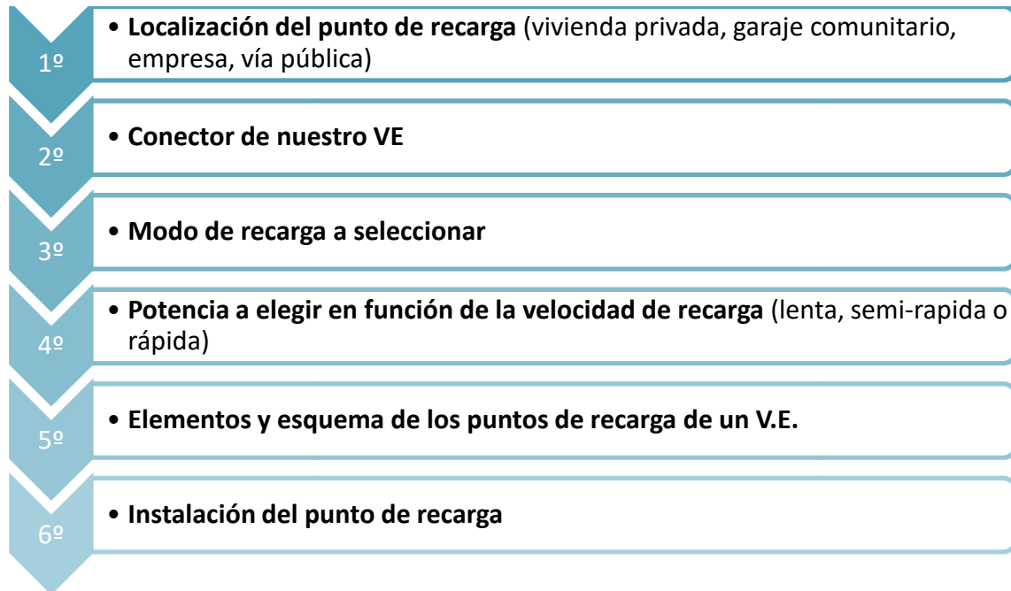
Figura 23. Esquema de pasos para la selección e instalación de un punto de recarga
