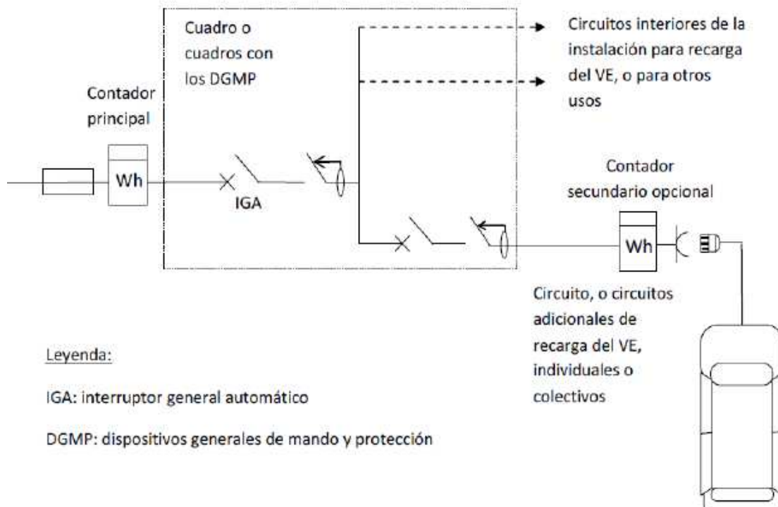
Figura 45. Esquema 4b: instalación con circuito o circuitos adicionales para la recarga del VEHÍCULO ELÉCTRICO [37]
